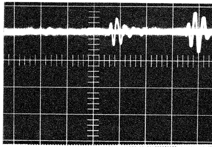
Bild 2. Oszillogramm der Freßgeräusche von Karpfen; unten am Rand eine auf demselben Tonband aufgezeichnete Vergleichsfrequenz
