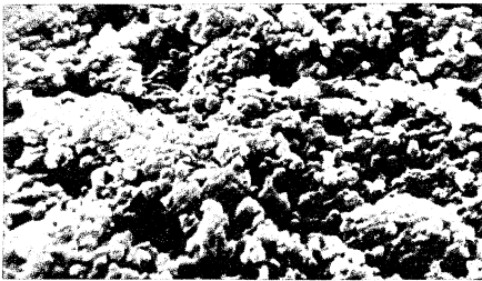
Bild 3. Aufnahme mit Hilfe eines Elektronenmikroskops der chemisch aufgerauhten Oberfläche des Haftvermittlers. Vergrößerung: etwa 13 000-fach (Aufnahme: Schering AG)
