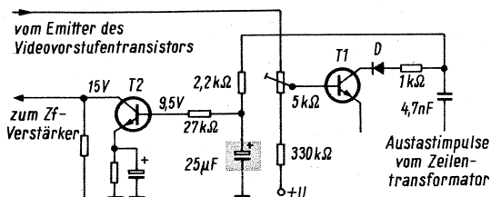
Vereinfachte Schaltung der Regelspannungserzeugung
