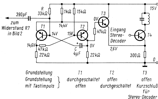
Bild 3. Monostabiler Multivibrator zum Stummtesten des Empfanges beim Betätigen der Fingertipp-Elektronik
