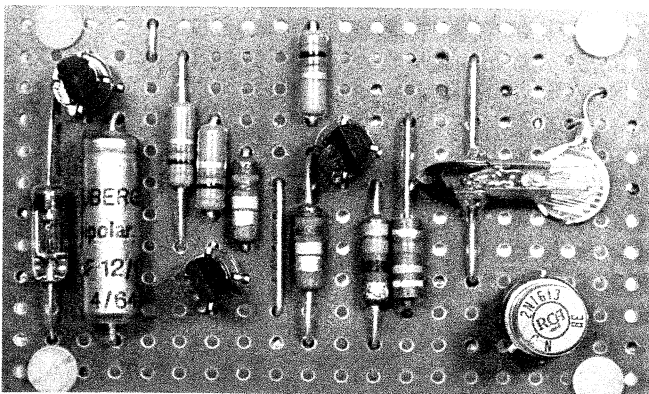
Bild 6. Aufbau des Schaltverstärker-Bausteines
