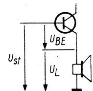
Bild 16. Emitterfolger. Die Steuerspannung ist gleich der Summe ( U_{BE} + U_L ), also starke Gegengekopplung durch den Spannungsabfall am Lastwiderstand
