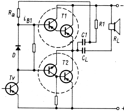
Bild 8. Ansteuerung mit komplementären Treibertransistoren
