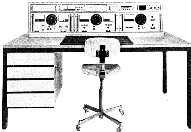
hera-Arbeits-tisch MK 1800 mit Unterbau MHG 49 mit LEP-Meß- und Prüfaufbau im Einschubsystem Fordern Sie Unterlagen!
