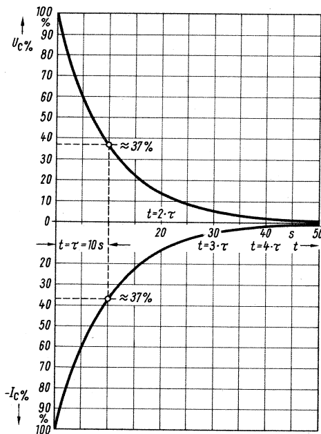
Bild 3.7. Entladekurven des Kondensators (Schaltung 3.5)
