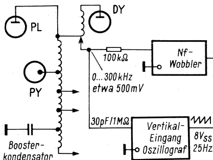
Bild 3. Blockschaltbild zur Aufnahme der Resonanzkurven gemäß Bild 1, 2, 4, 5, 6
