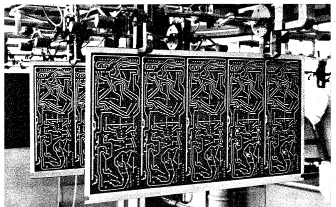
Bild 5. Fertig bearbeiteter Zuschnitt nach der chemisch-galvanischen Behandlung: Basisschicht abgeätzt, Leiterbahn mit Pb-Sn-Auflage
