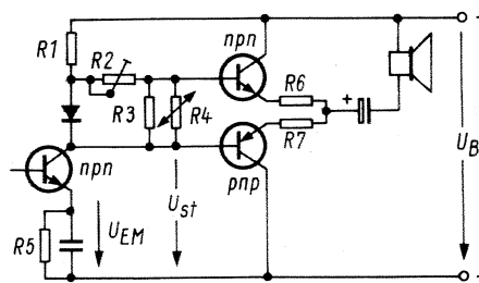
Bild 15. Schaltung für eine komplementäre Endstufe
