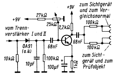
Bild 13. Misch- und Differenzfrequenz-Verstärkerstufe zu Bild 9
