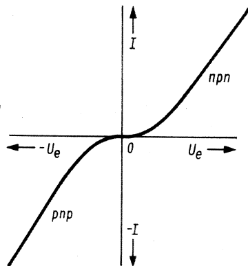
Bild 13. Kennlinienverlauf, wenn die Eingänge der beiden Endtransistoren gleichstrommäßig parallel geschaltet werden
