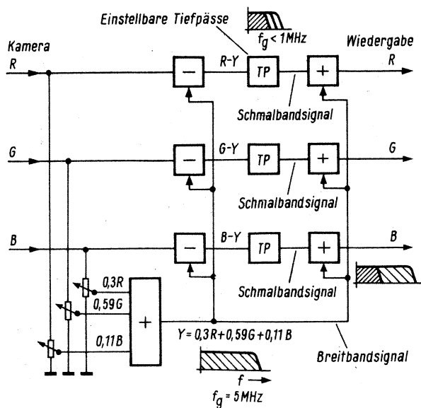
Bild 9 Bildung der Farbdifferenzsignale (R - Y), (G - Y) und (B - Y), ihre schmalbandige Übertragung und die Wiedersummensetzung zu R, G und B durch Addition des breitbandig übertragene Leuchtdichtesignales (Methode der „mixed highs“)
