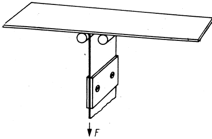
Bild 6. Prinzip der Prüfmaschine für die Haftfestigkeit der Kupferfolie
