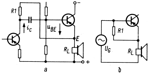
Bild 17. Der Einfluß des Spannungsabfalls an R_L auf die Basis-Emitterspannung. a = bei hochohmigem Signalgenerator (Treiberstufe), b = bei niederohmigem Signalgenerator
